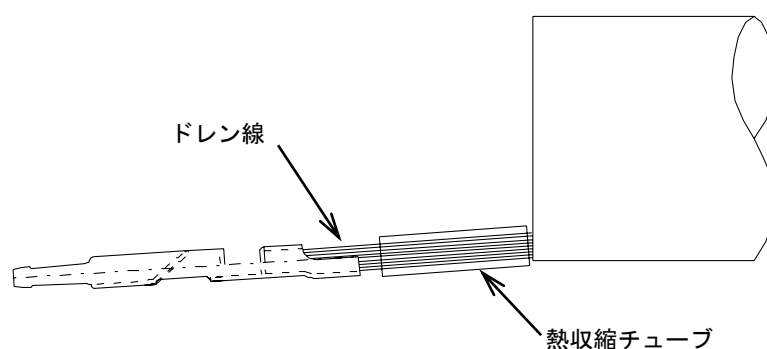
ドレン線はんだ付けの場合
