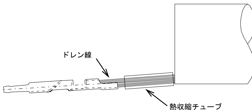
ドレン線をはんだ付けの場合
