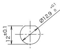
パネル取付穴参考寸法
