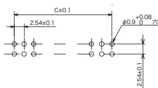
プリント基板取付参考寸法図
