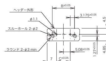
プリント基板取付寸法図
