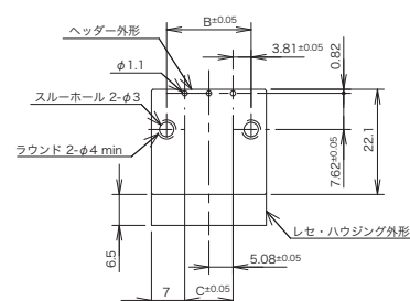
プリント基板取付寸法図
