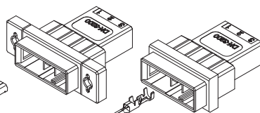
タブコンタクト
