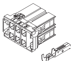
レセプタクルコンタクト
