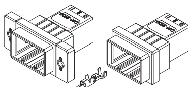
タブコンタクト
