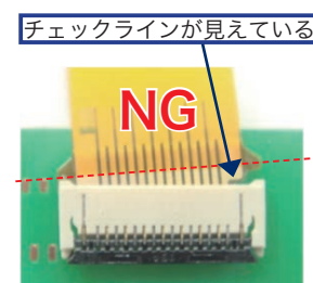
写真⑧：斜め挿入状態
