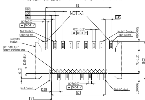
品 名 芯 数 A B C D E FF52-8A-R11A-3J 8 4.60 3.00 2.10 3.55 3.50 FF52-15A-R11A-3J 15 6.70 5.10 4.20 5.65 5.60 FF52-17A-R11A-3J 17 7.30 5.70 4.80 6.25 6.20 FF52-19A-R11A-3J 19 7.90 6.30 5.40 6.85 6.80
