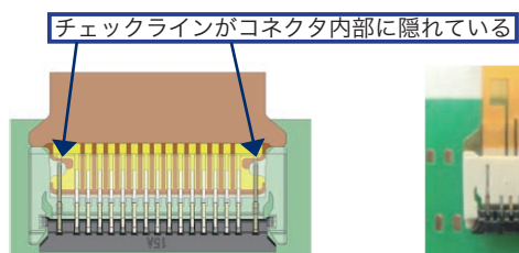
図⑥：正常挿入状態
