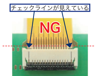
写真⑦：浅挿入状態
